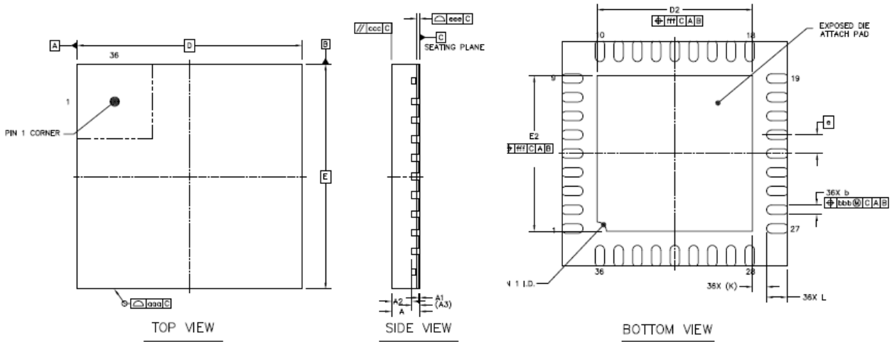
图 27QFN36 封装图
